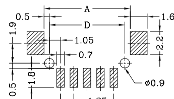
P.C.B LAYOUT 线路板布局图
