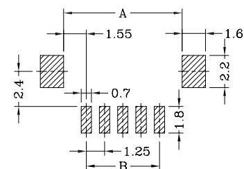
P.C.B LAYOUT 线路板布局图
