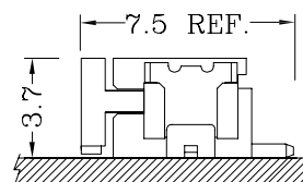
SMR-Type/卧贴型
