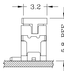
SMS-Type/立贴型
