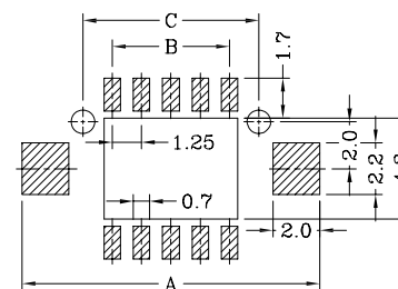
P.C.B LAYOUT 线路板布局图
