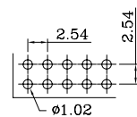
PCB LAYOUT 线路板布局图
