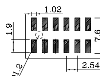
PCB LAYOUT 线路板布局图
